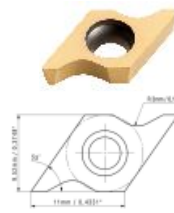
CARBIDE INDEXABLE INSERTS R3
